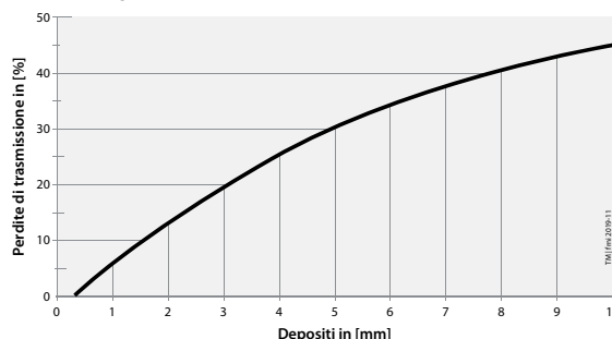
Perdita di potenza in % a causa di incrostazioni calcaree
