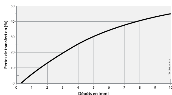
Perte de puissance en % due au dépôt calcaire
