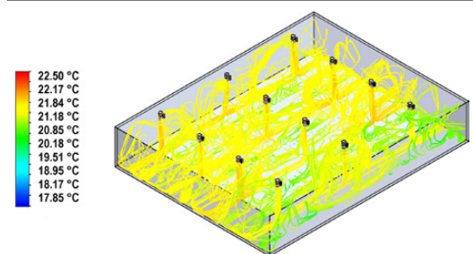
Simulacije raspodjele temperature omogućuju preciznije planiranje i projektiranje.
