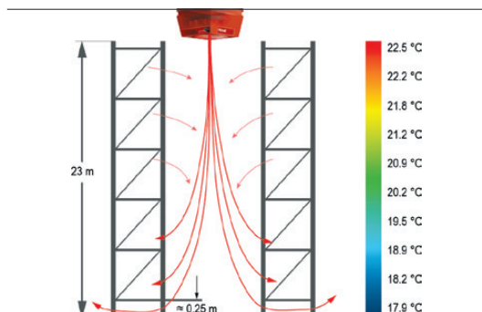
Temperaturna stratifikacija svedena je na minimum zahvaljujući distribuciji zraka s Hoval Air-Injector-om.
